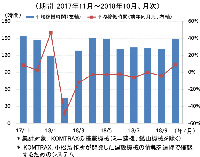
図表2. 小松製作所製建設機械の中国地域稼働時間 (一台当たり月間平均稼働時間)
