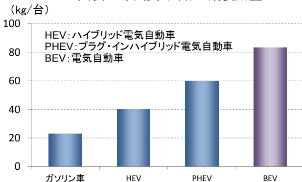
図表3. 自動車(1台)の銅使用量
